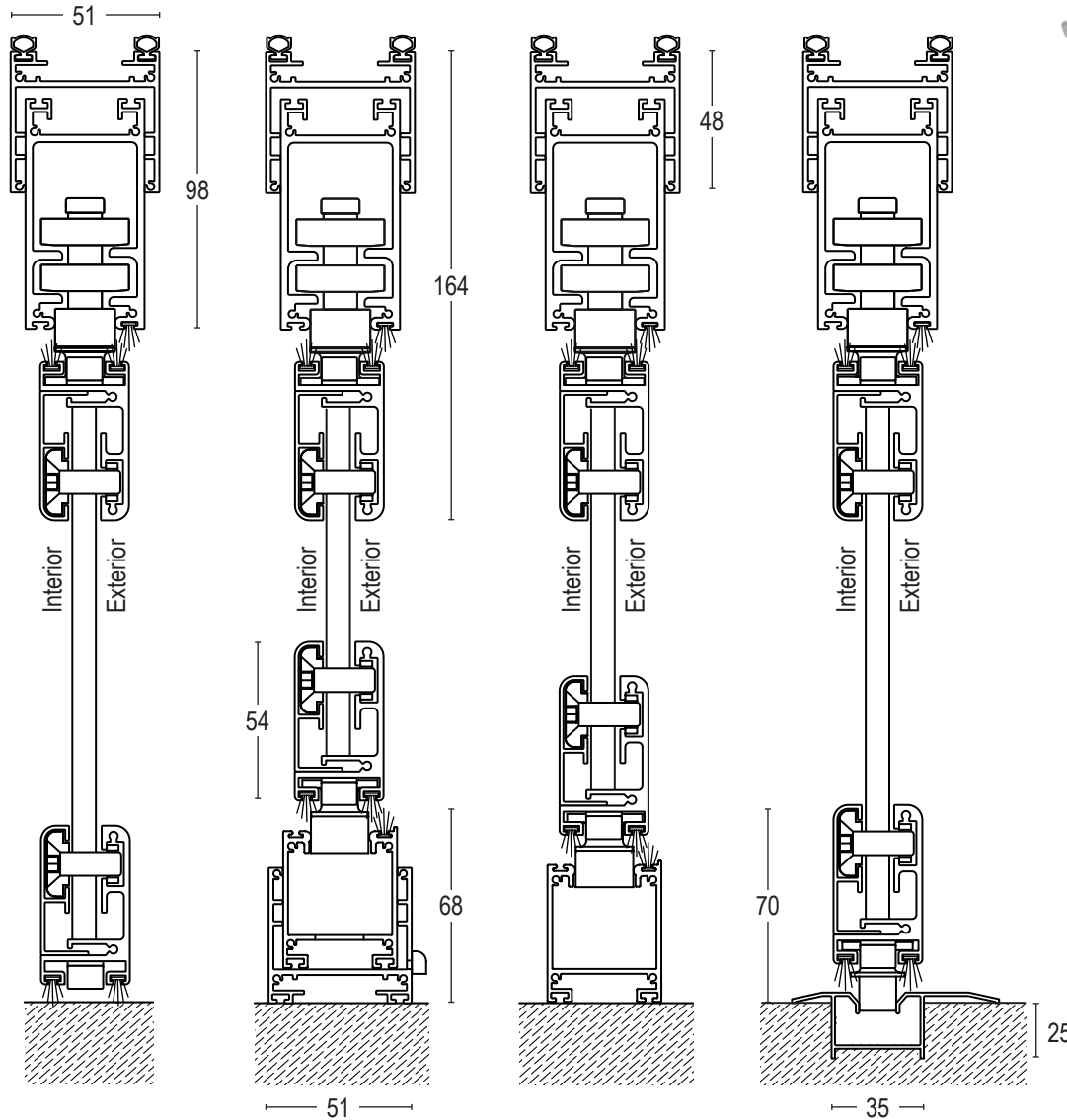
Sin guía inferior
