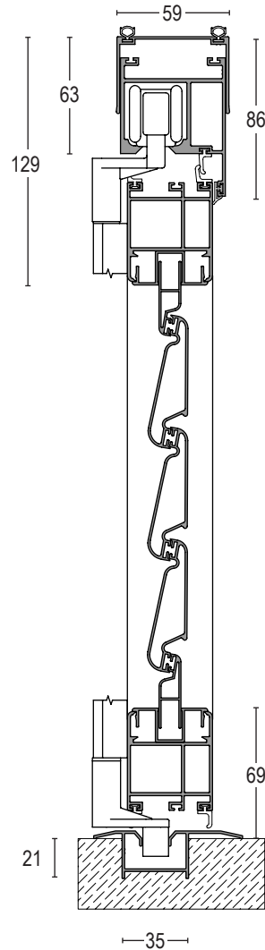
Cadre inférieur encastré
