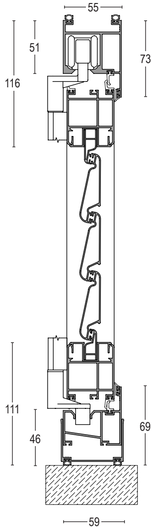
Cadre inférieur superposé
